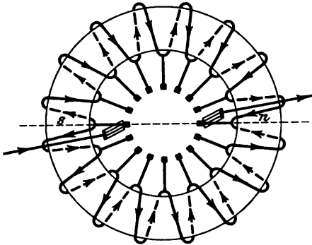
Abb. 137. Geschlossene Ringwicklung mit Stromzuführung an zwei gegenüberliegenden Stellen.
